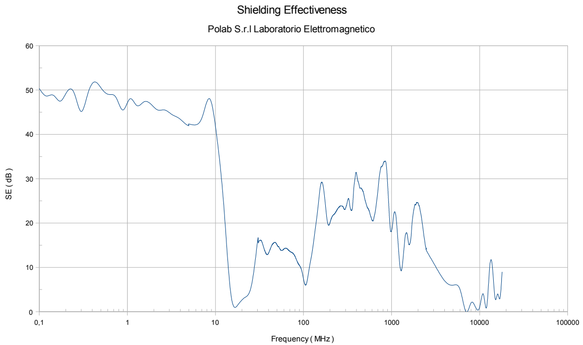
Figura 1 Grafico dell'efficacia di schermatura ( campo elettrico ed onda piana )
